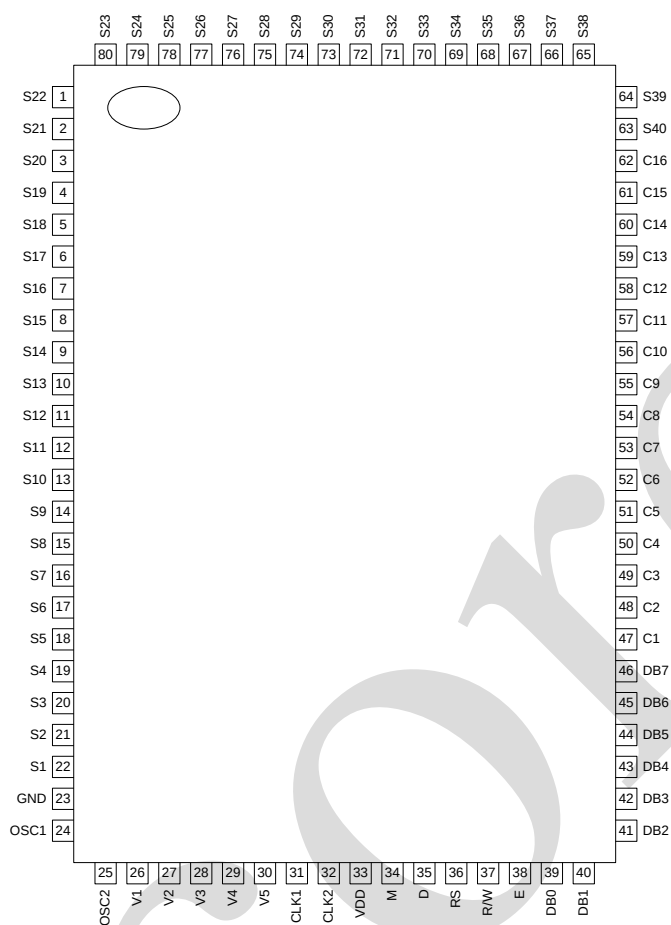
QFP80
