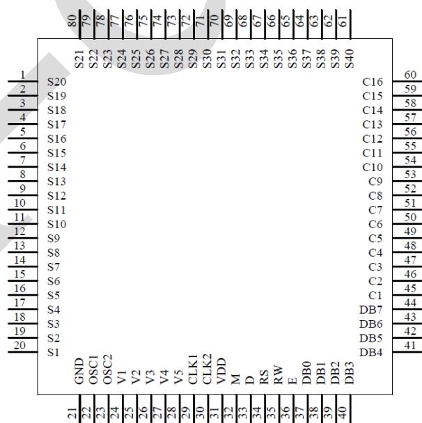
LQFP80
