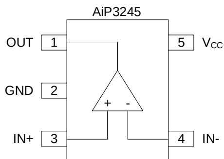
SOT23-5/SOT353
