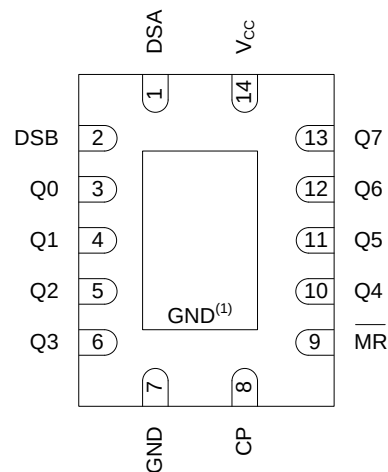
DHVQFN14
