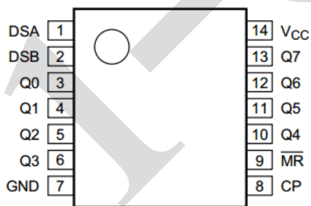
DIP14/SOP14/TSSOP14
